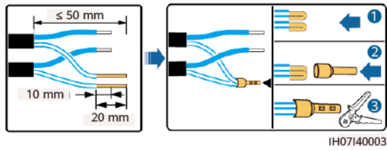
Figura 5-25 Crimpagem de dois cabos de sinal
