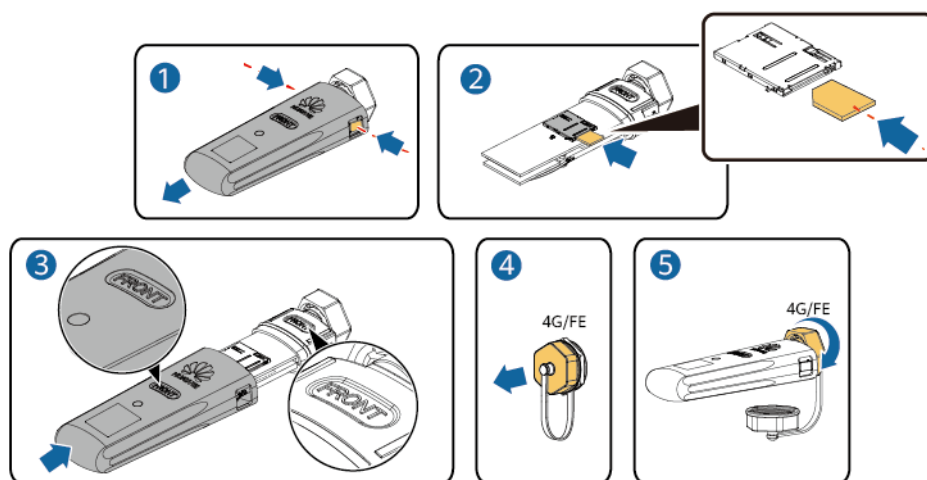
Figura 5-4 Instalação do 4G Smart Dongle
