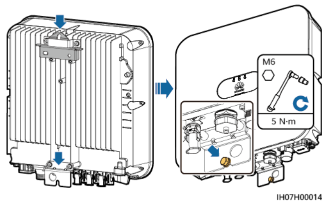
Figura 4-17 Aperto dos conjuntos de parafusos
