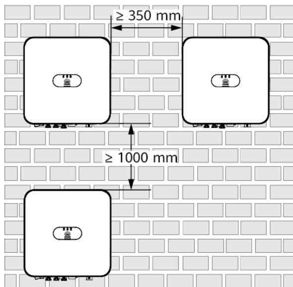
Figura 4-5 Instalação sobreposta (não recomendada)
