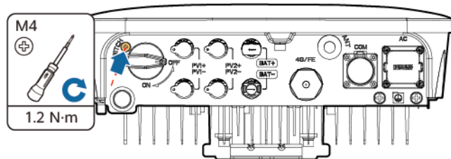
Figura 4-10 Instalação de um parafuso de travamento na DC switch
